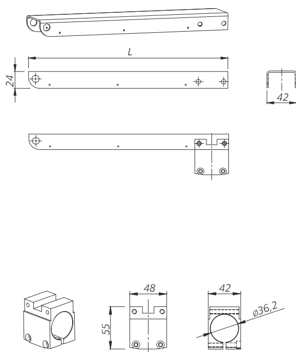
Rys. 110 Konsola przesuwna do montażu siłownika wrzecionowego typ S z przesuniętym punktem obrotu na oknie oddymiającym, wymiary [mm]
