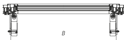
Rys. 29 Przekrój poziomy B-B przez okno oddymiające mcr OSO THERM 75 z przesuniętym punktem obrotu w pozycji zamkniętej
