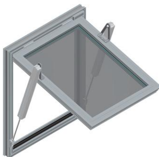
Rys. 56 Okno oddymiające mcr OSO THERM 75 z dwoma sióownikami wrzecionowymi G
