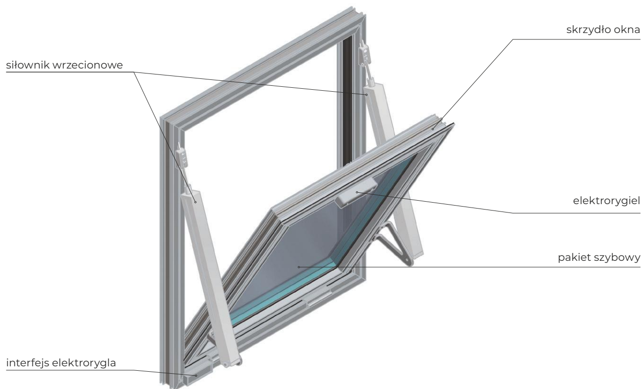
Rys. 62 Okno oddymiające mcr OSO THERM 75 otwierane do wewnątrz za pomocą dwóch siłowników wrzecionowych z elektrotrygiel i interfejsem
