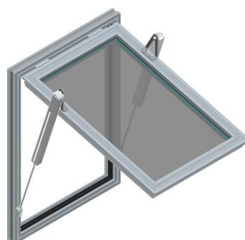
Rys. 90 Okno oddymiające mcr OSO THERM 75 z dwoma siłownikami wrzecionowymi G z przesuniętym punktem obrotu
