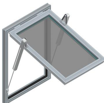
Rys. 59 Okno oddymiające mcr OSO THERM 75 z dwoma sióownikami wrzecionowymi G z przesuniętym punktem obrotu
