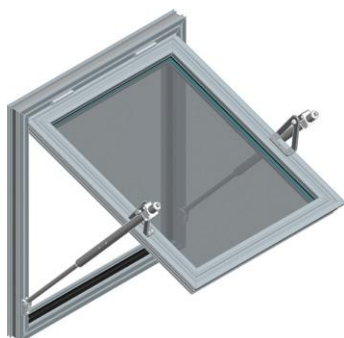
Rys. 58 Okno oddymiające mcr OSO THERM 75 z dwoma sióownikami wrzecionowymi S z przesuniętym punktem obrotu
