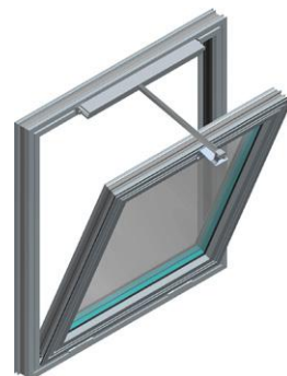
Rys. 51 Okno oddymiające mcr OSO THERM 75 z sióownikiem łańcuchowym HCV
